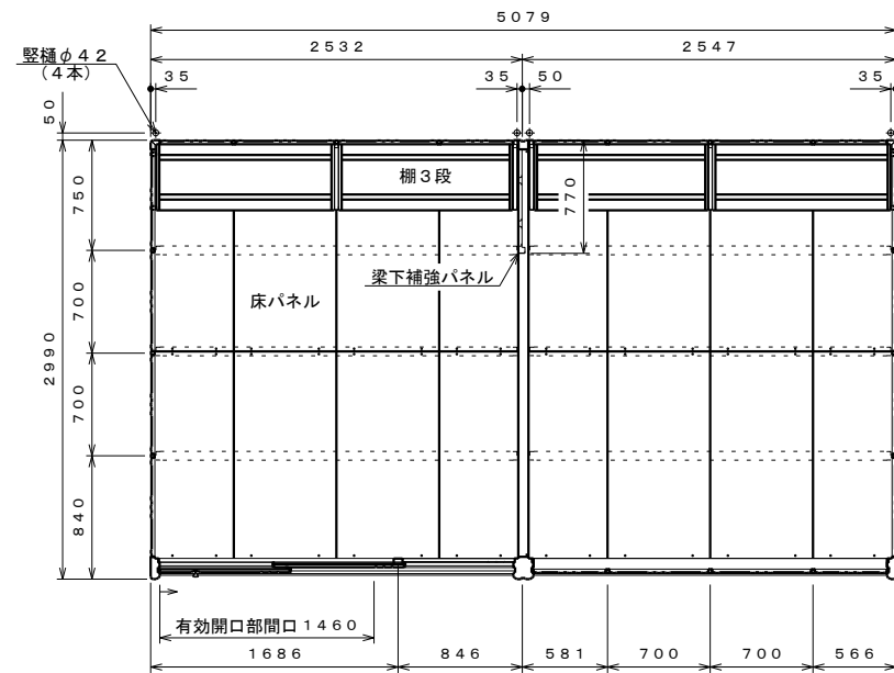
平面図 S=1:40
