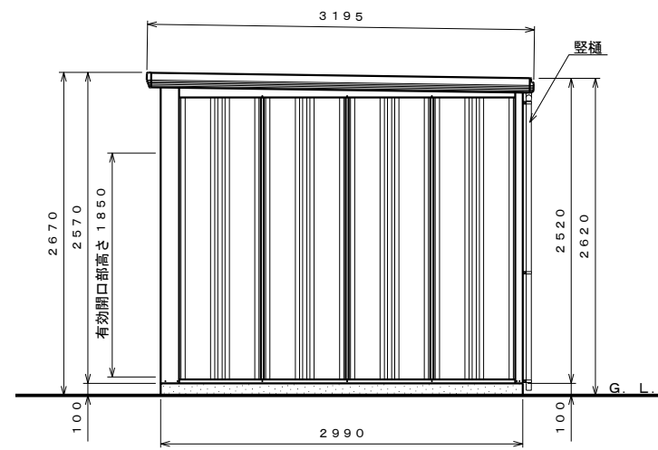
側面図 S=1:40
