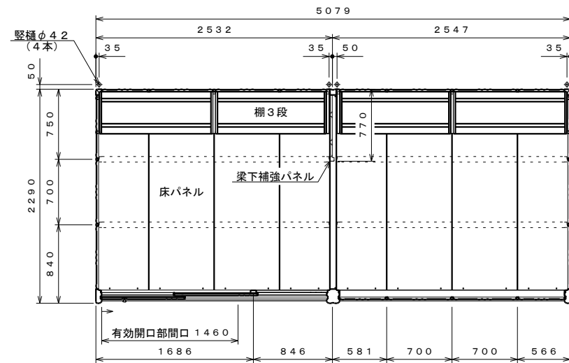
平面図 S=1:40
