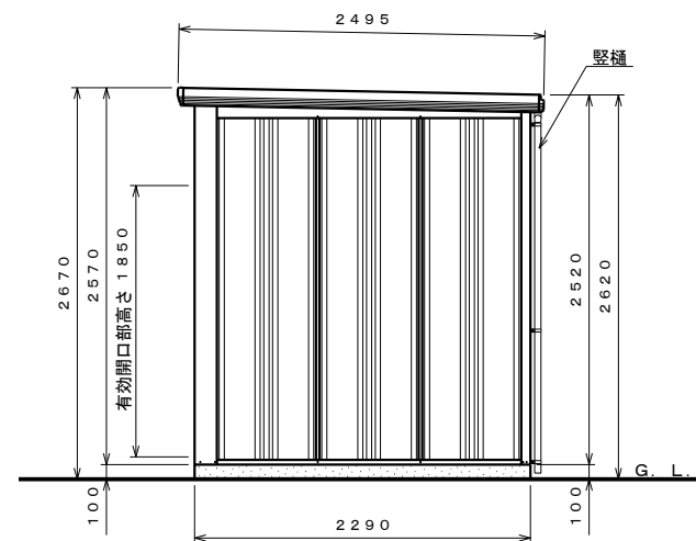
側面図 S=1:40
