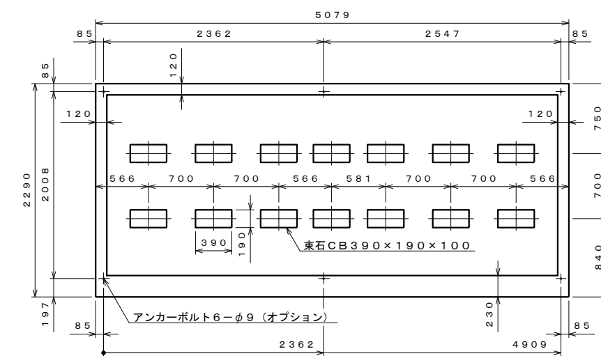
基礎伏せ図 S=1:40
