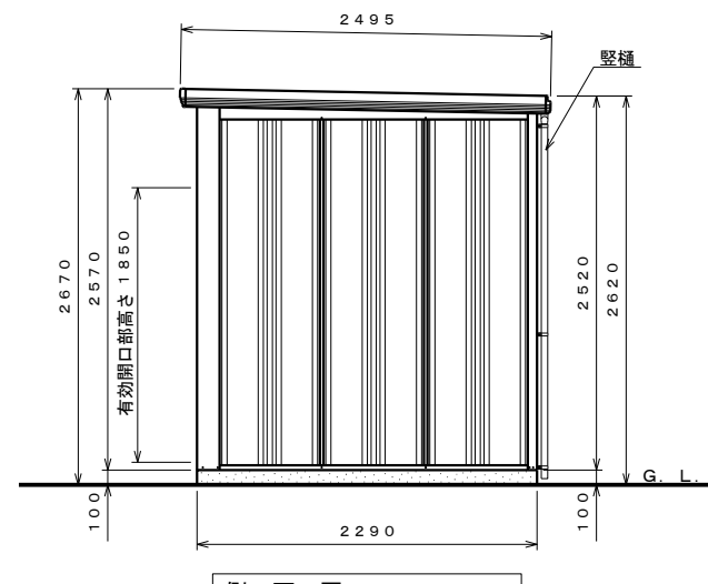
側面図 S=1:40
