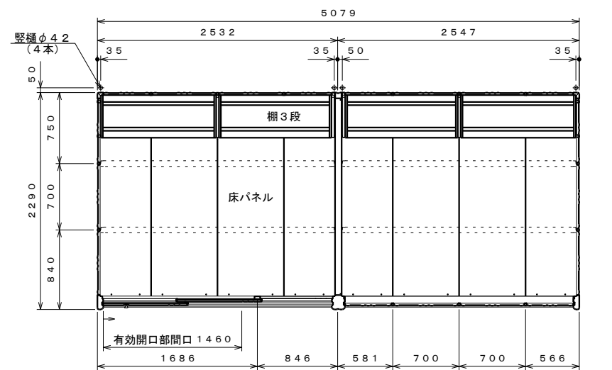
平面図 S=1:40
