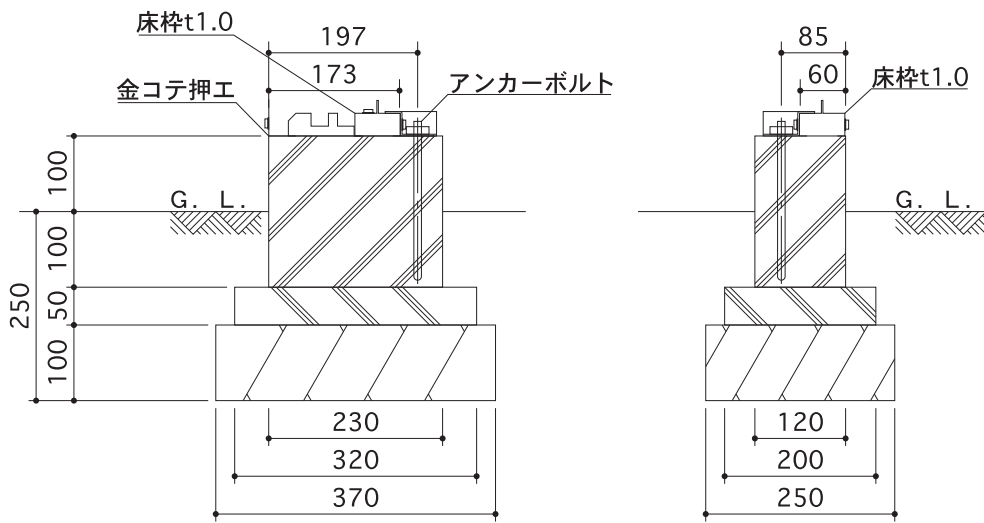
A-A断面図
