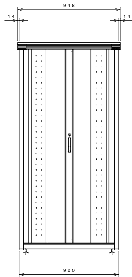
正面図
