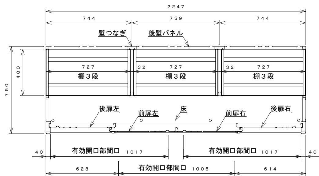
平面断面図
