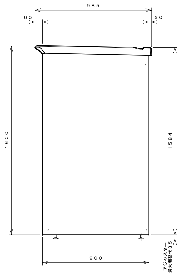
右側面図
