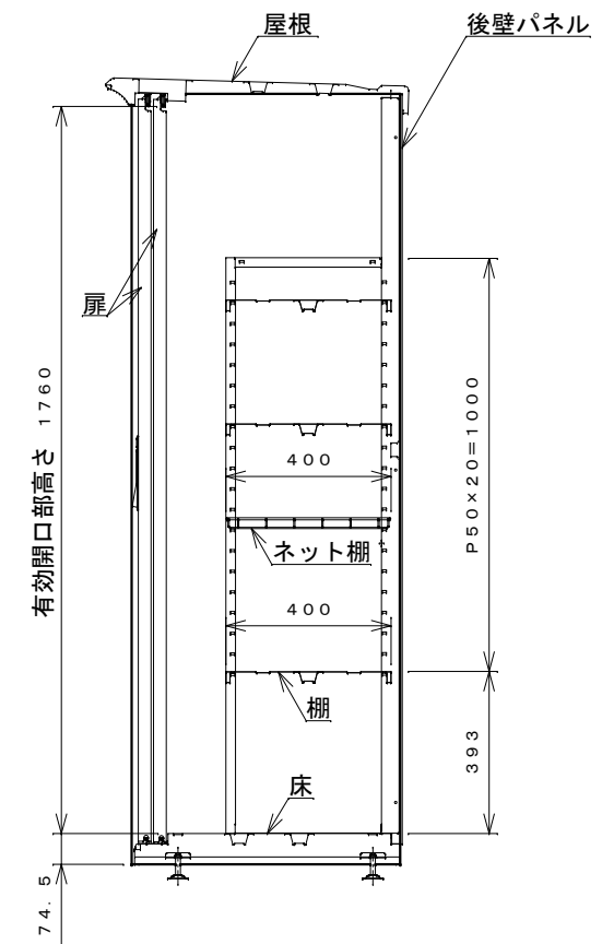
側面断面図
