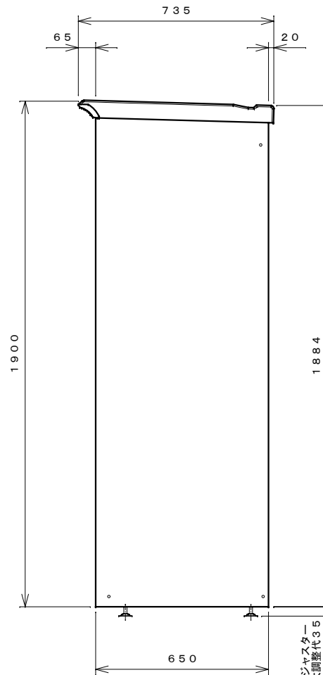
右側面図
