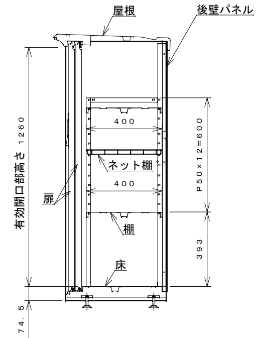
側面断面図
