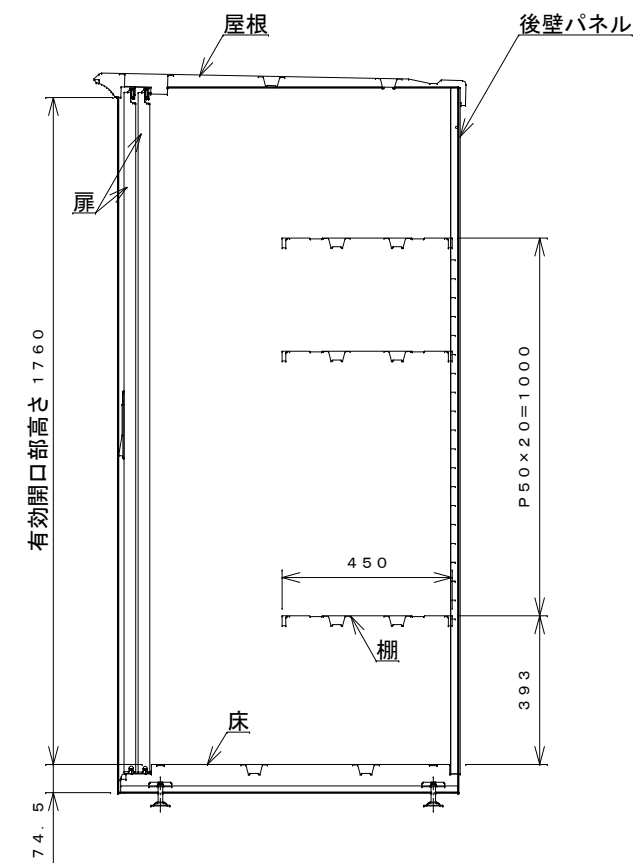
側面断面図
