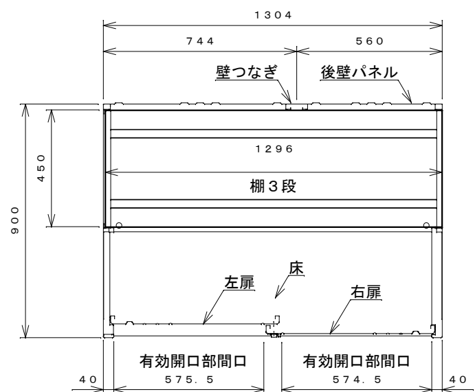
平面断面図
