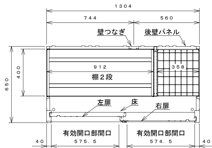
平面断面図
