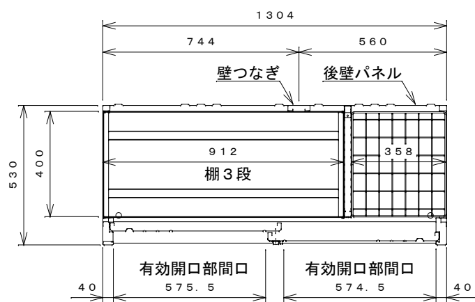
平面断面図
