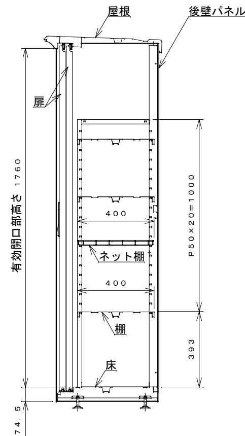
側面断面図
