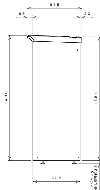
右側面図
