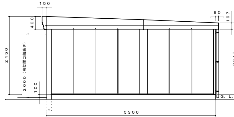
側面図 S=1:50
