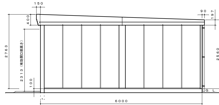
側面図 S=1:50
