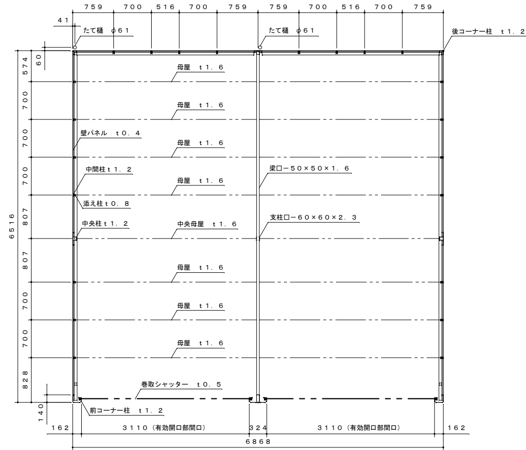
平面図 S=1:50
