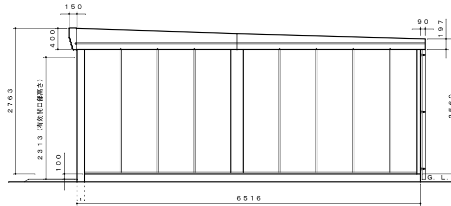
側面図 S=1:50
