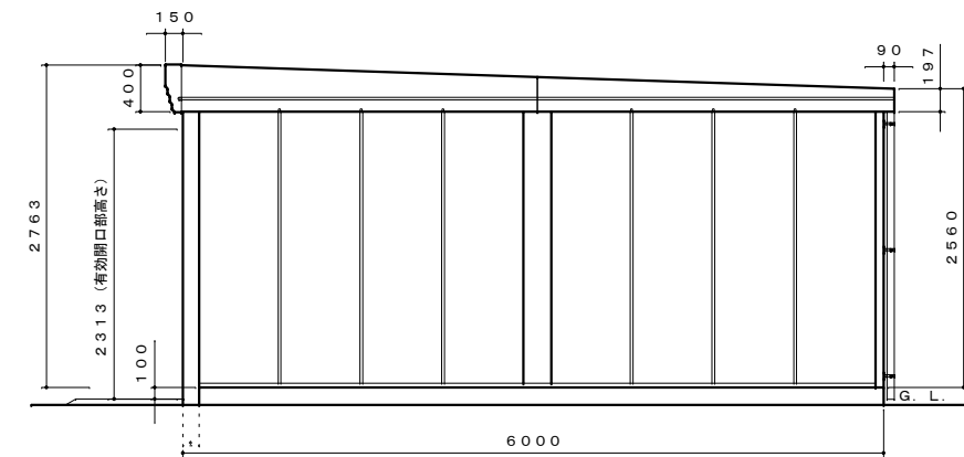
側面図 S=1:50
