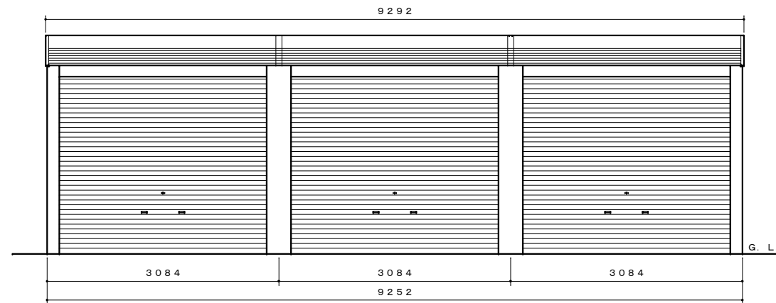
正面図 S=1:50
