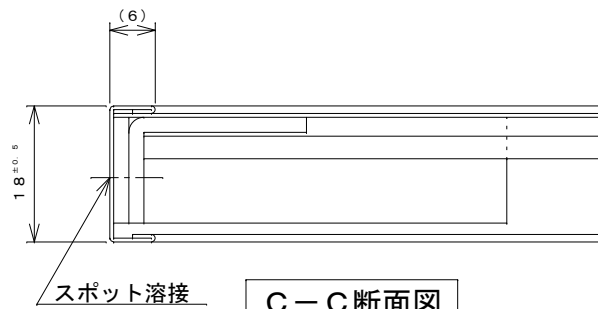
C-C断面図 S=1:1
