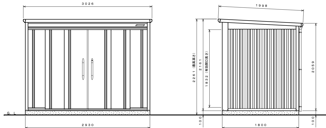
正面図 S=1:30
