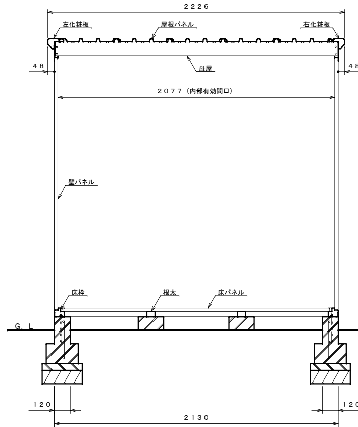
正面断面図 S=1:20
