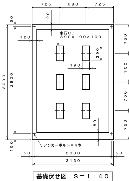
平面図 S=1:40
