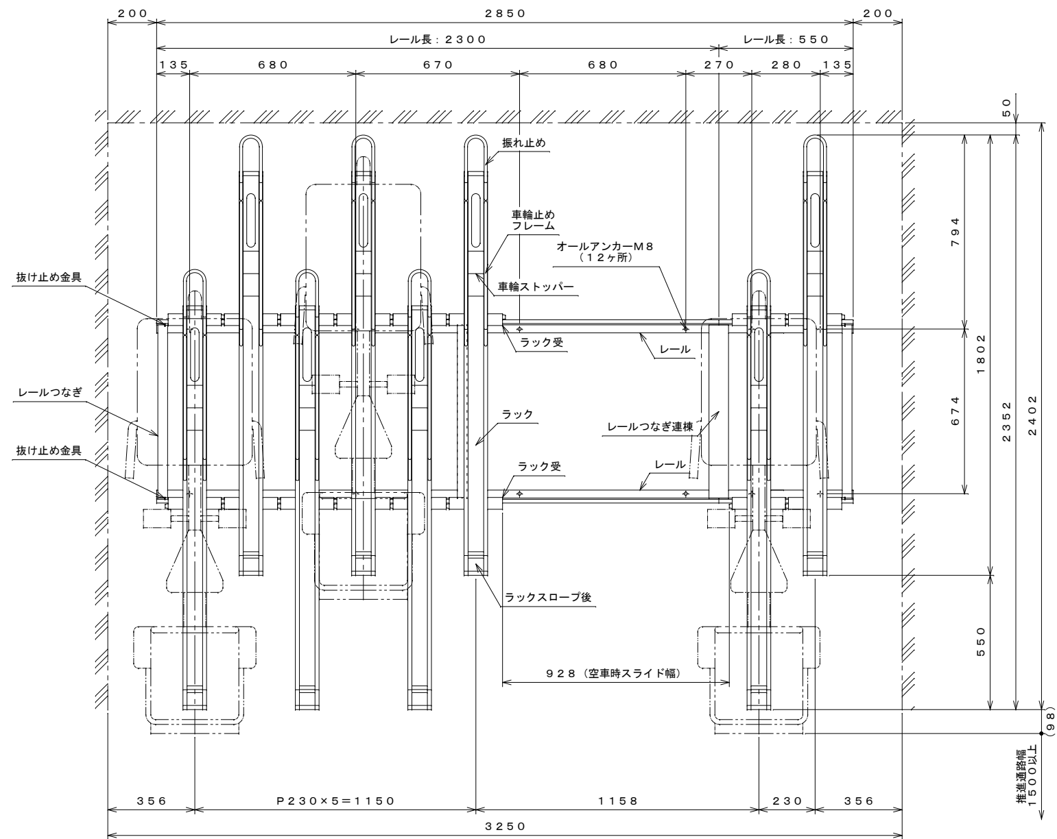
平面図 S=1:15
