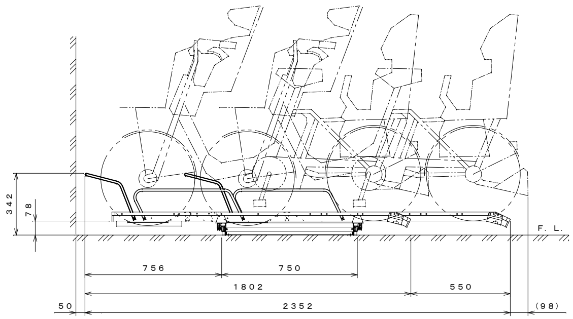
側面図 S=1:15
