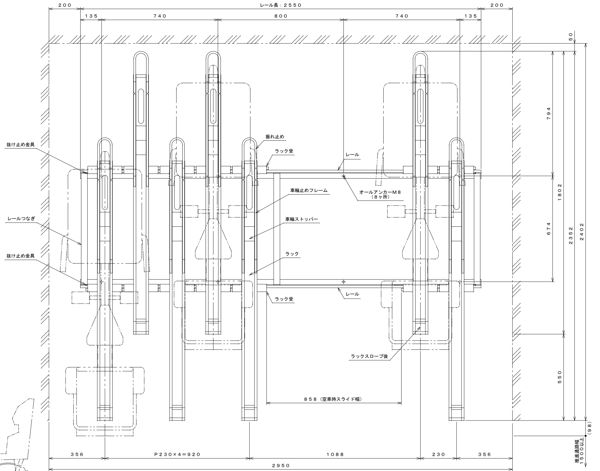
平面図 S=1:10
