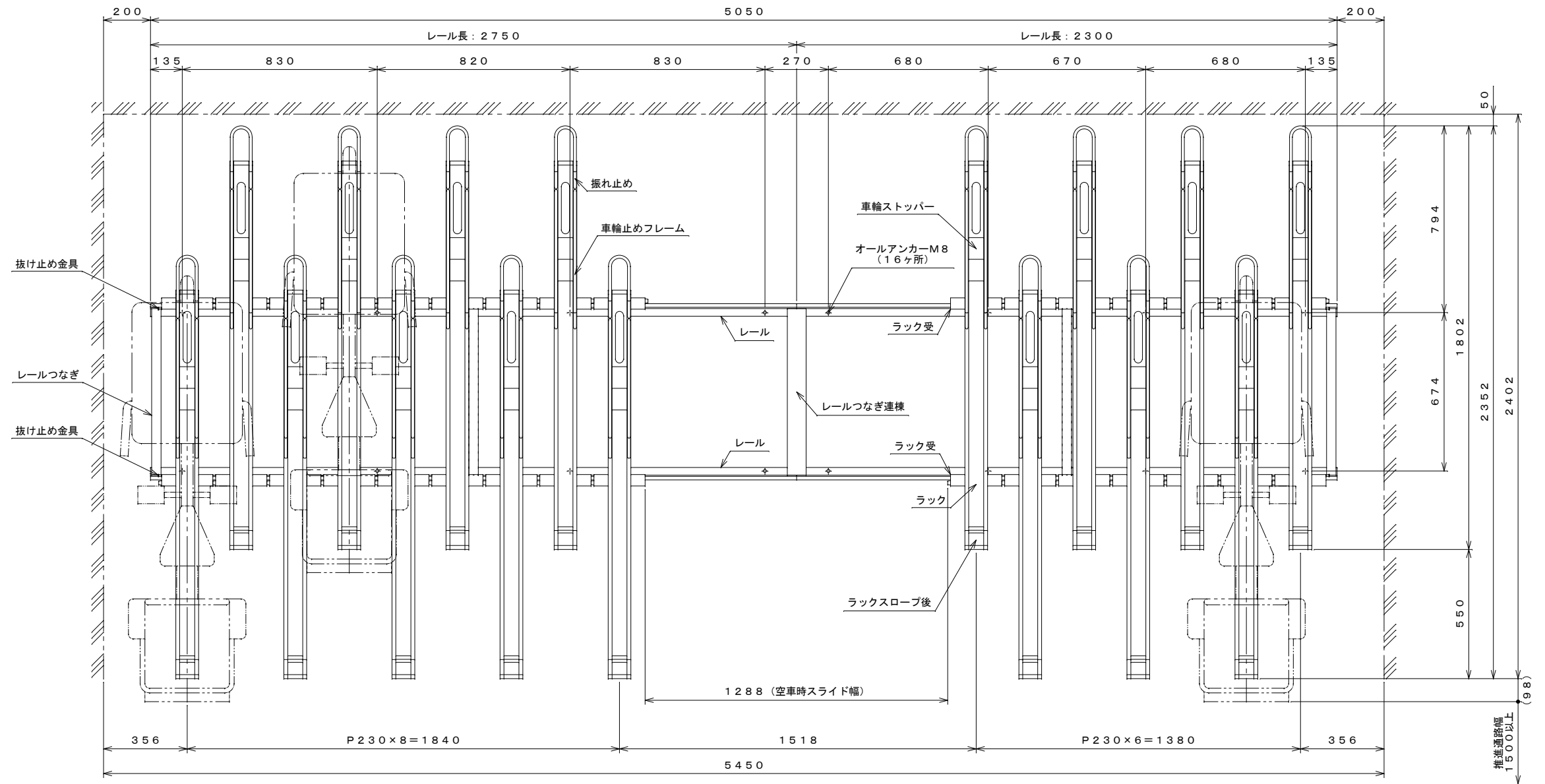
平面図 S=1:15
