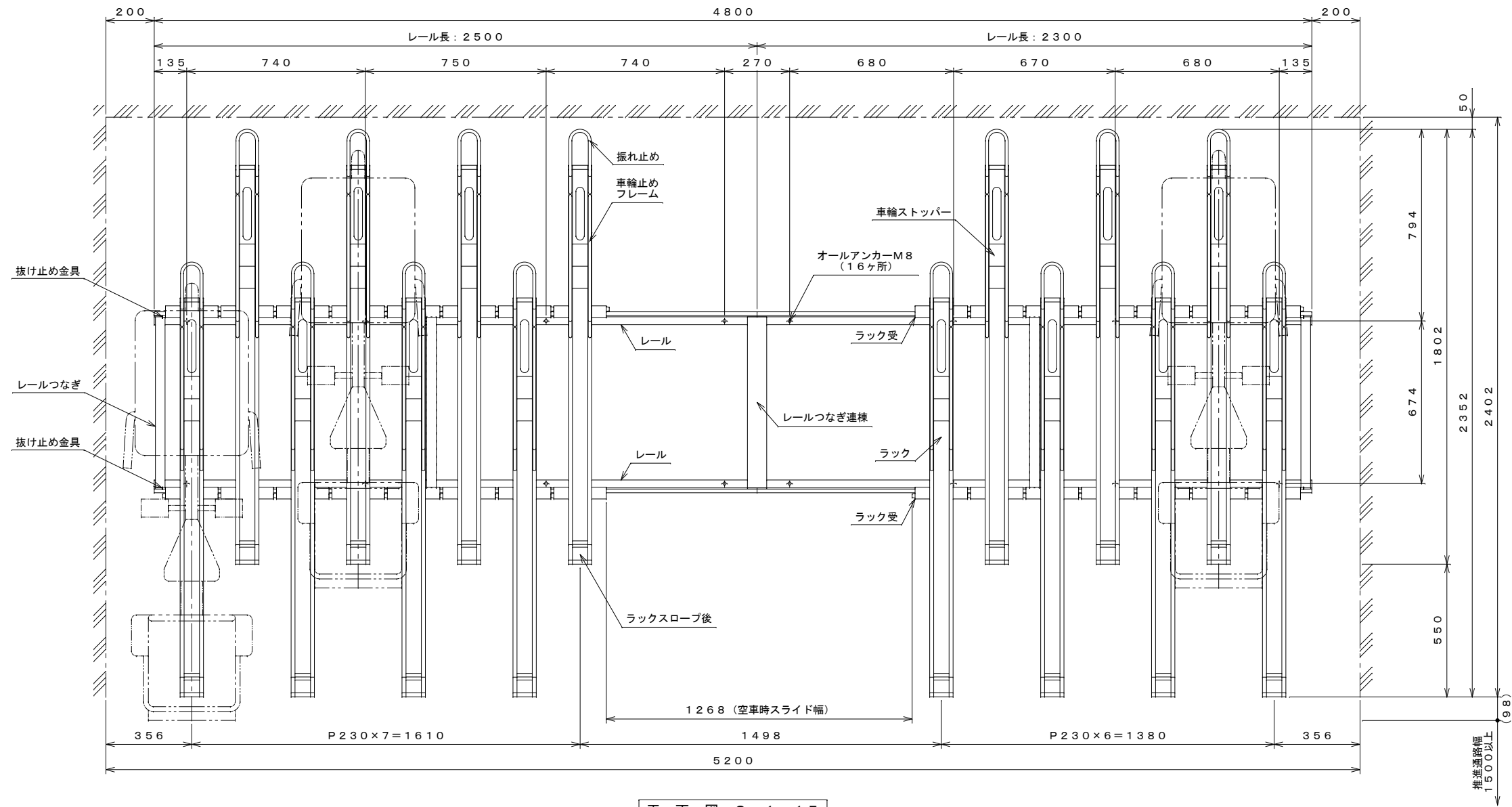
平面図 S=1:15
