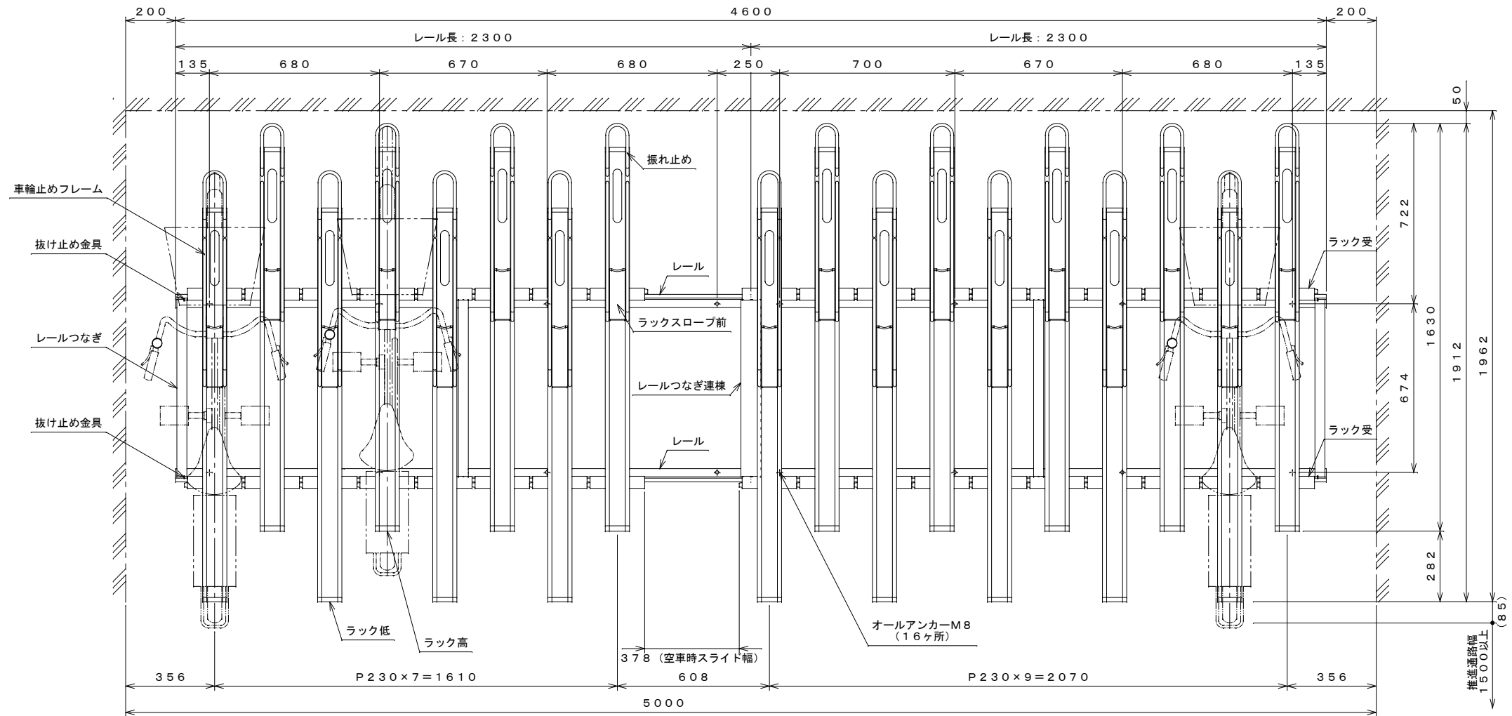
平面図 S=1:15
