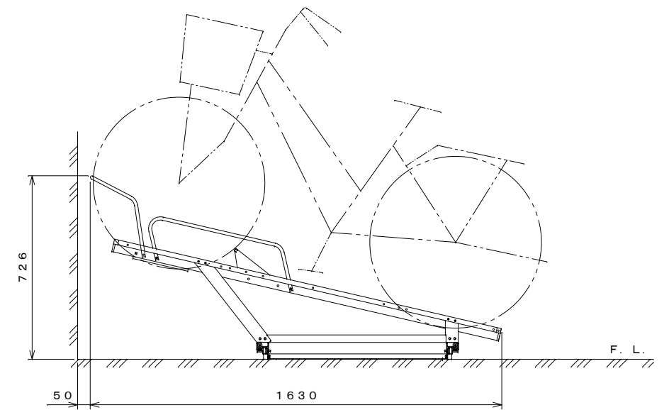
ラック高 側面断面図 S=1:15
