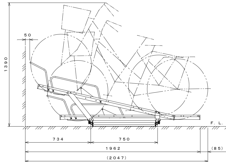
側面図 S=1:15
