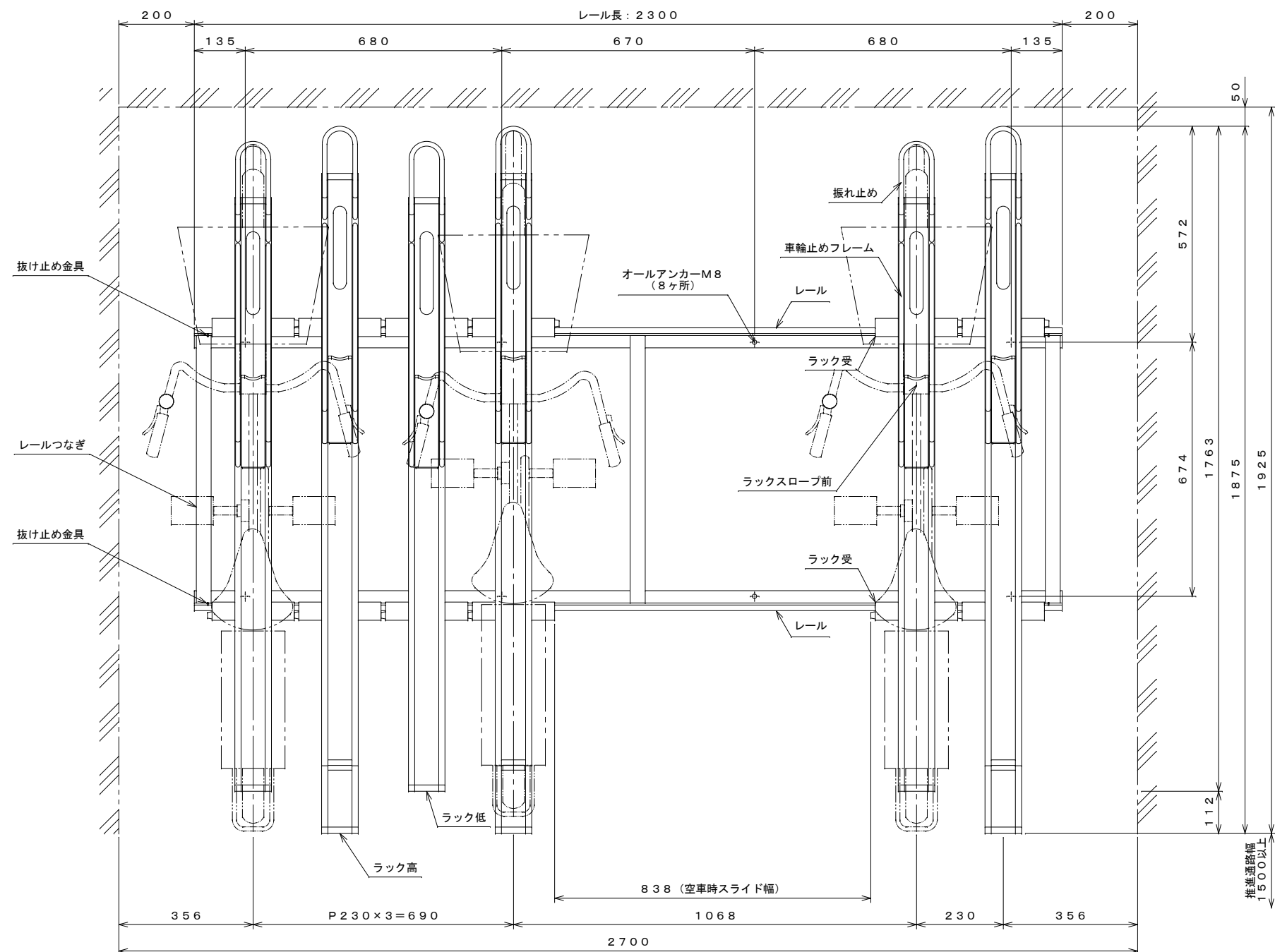
平面図 S=1:10
