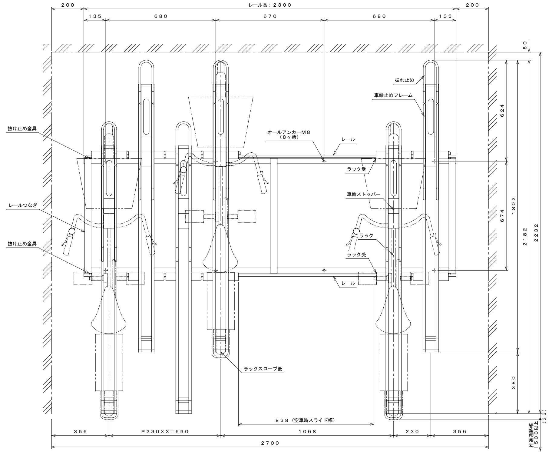
平面図 S=1:10
