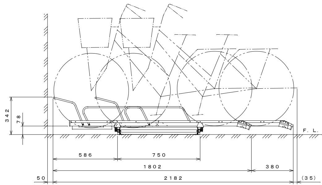
側面図 S=1:15
