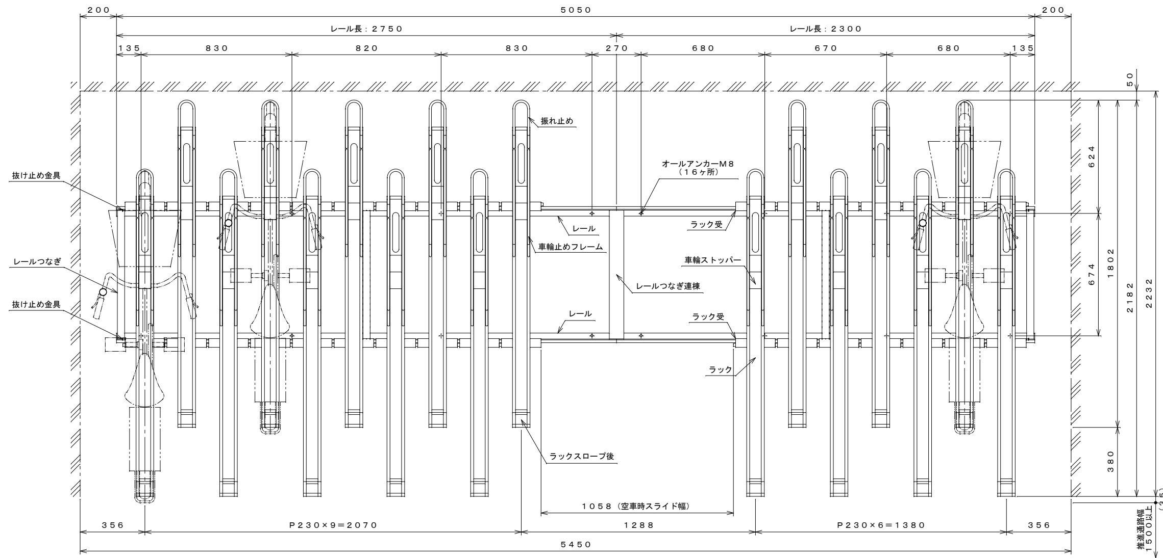
平面図 S=1:15
