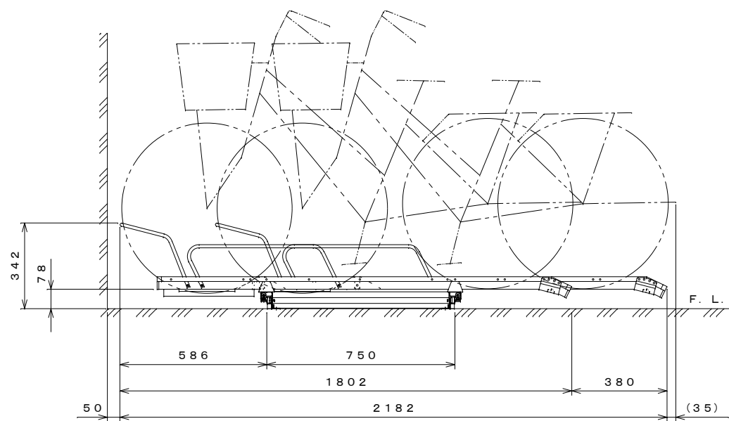
側面図 S=1:15
