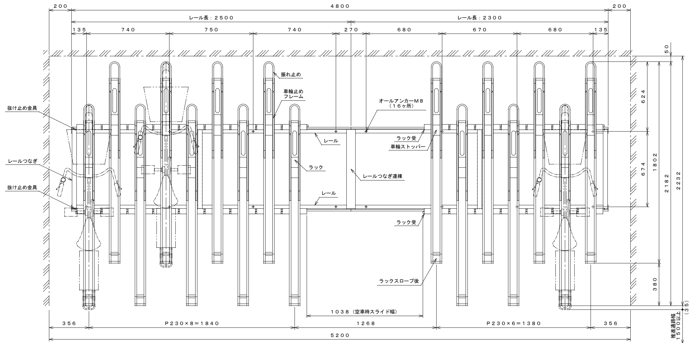
平面図 S=1:15
