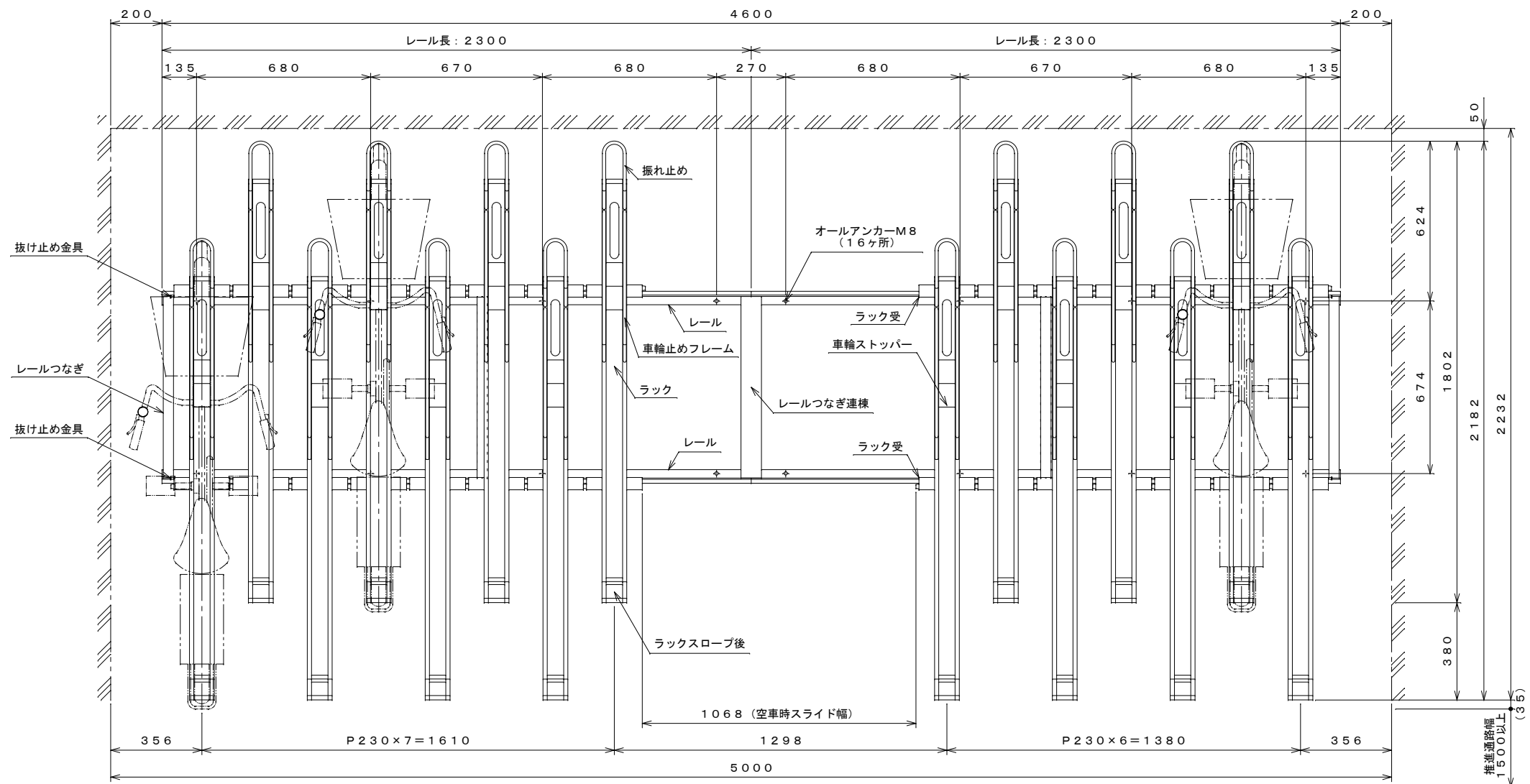
平面図 S=1:15
