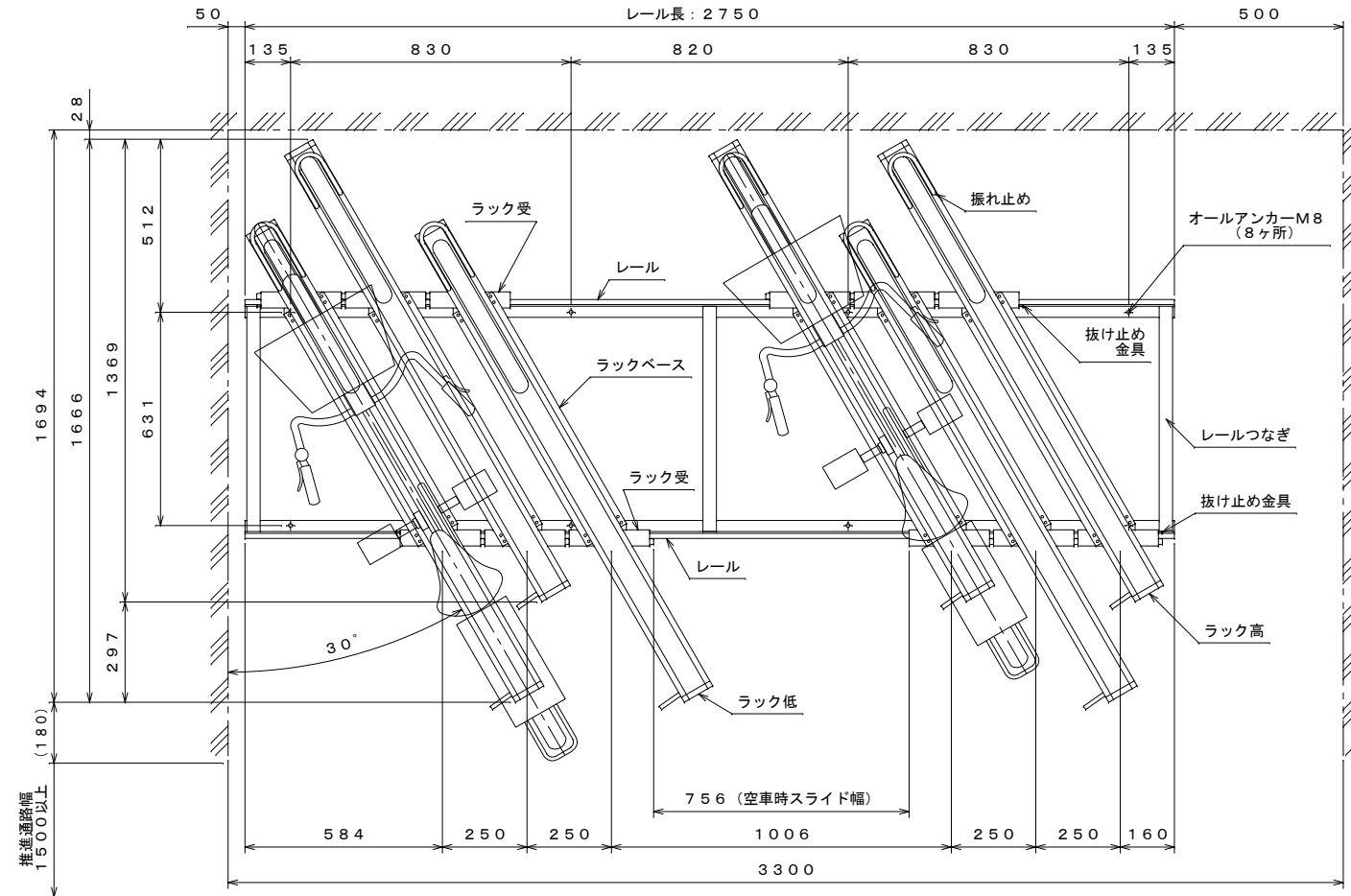
平面図 S=1:15
