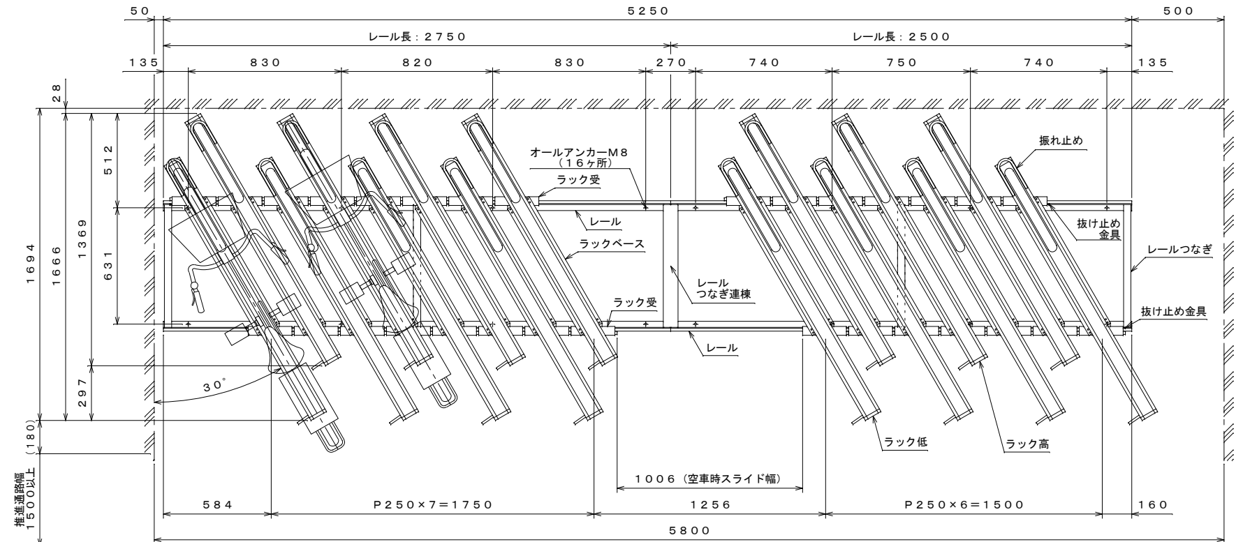
平面図 S=1:20
