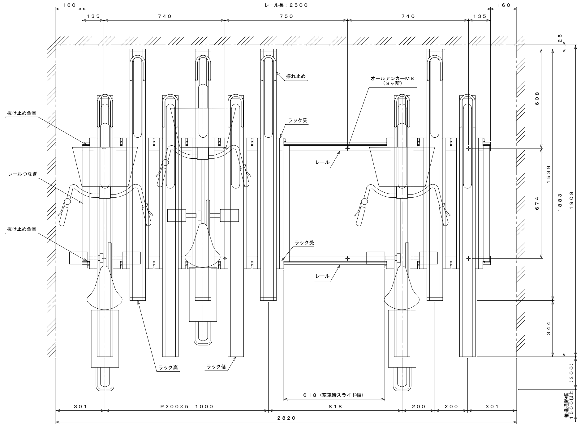
平面図 S=1:10
