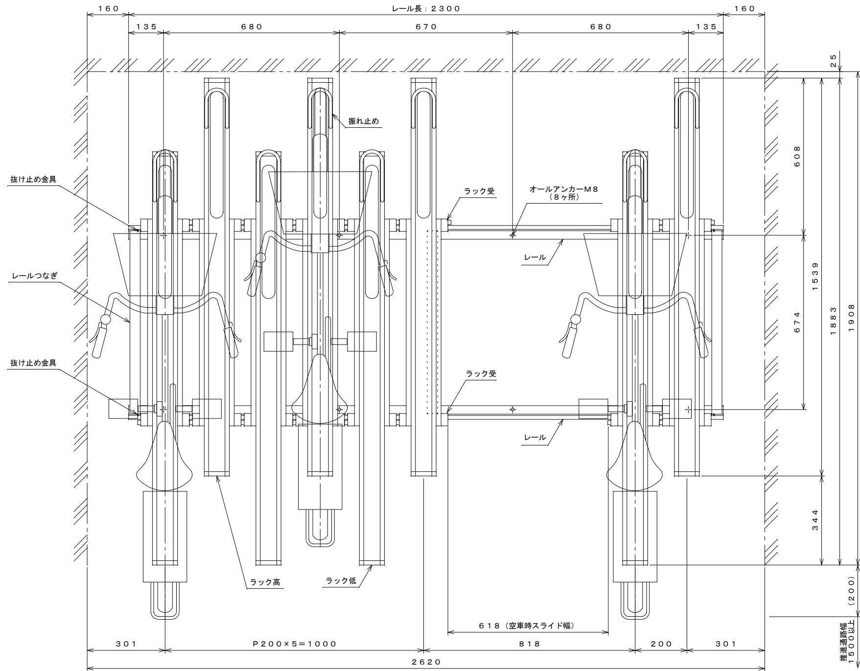
平面図 S=1:10
