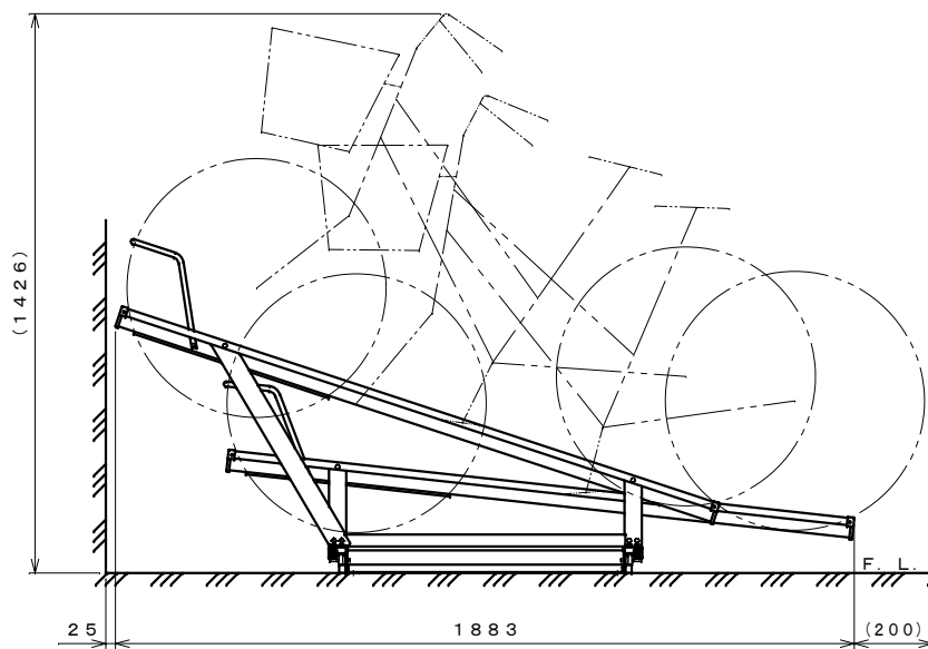
側面図 S=1:15
