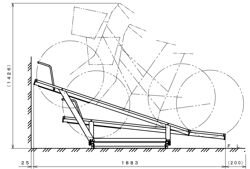
側面図 S=1:15
