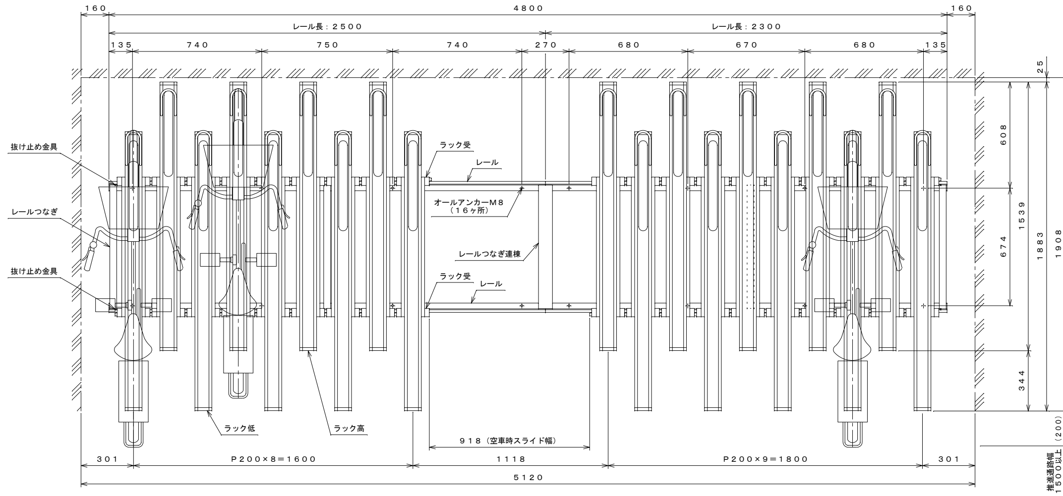
平面図 S=1:15
