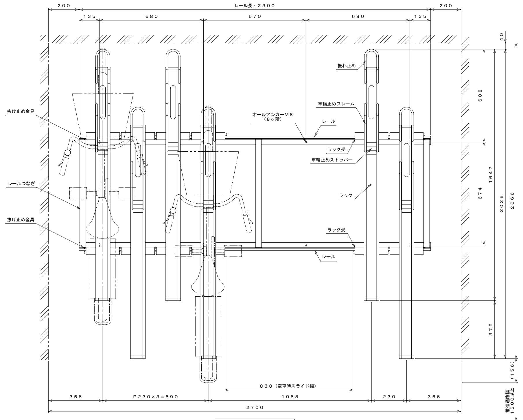
平面図 S=1:10
