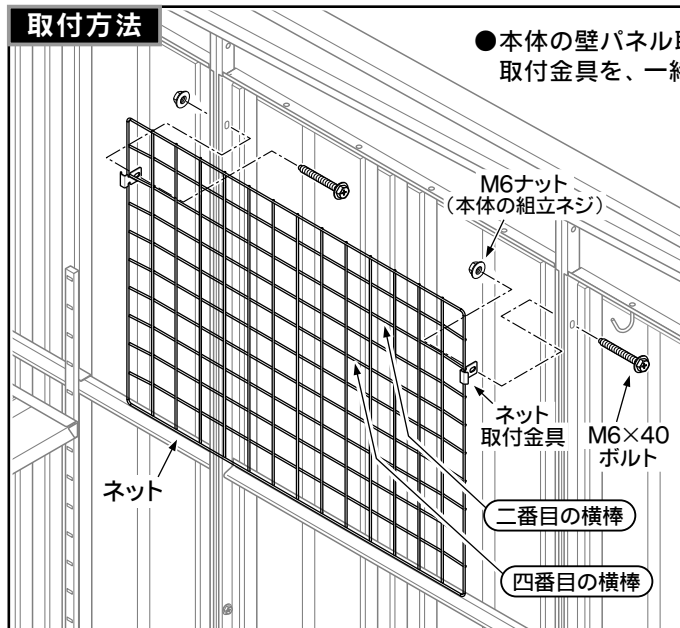
M6×40ボルト … 2本 (アブセットセムスM6×40棒先)
