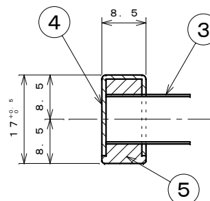
B-B断面図 S=1:1
