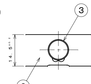
C-C断面図 S=1:1
