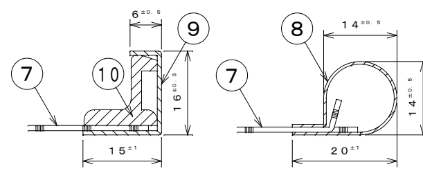
C-C断面図 S=1/1
