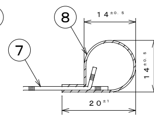
D-D断面図 S=1/1
