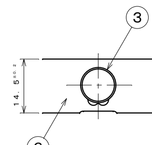
C-C断面図 S=1:1
