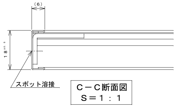
D部詳細図 S=1:1
