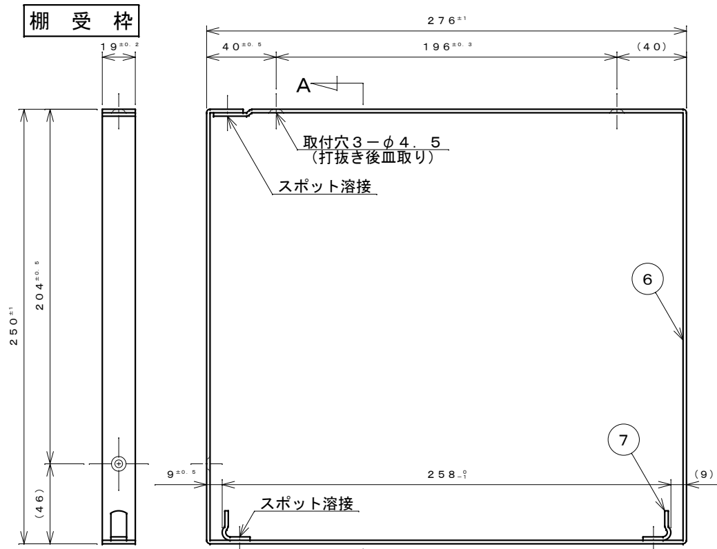
A-A断面図
