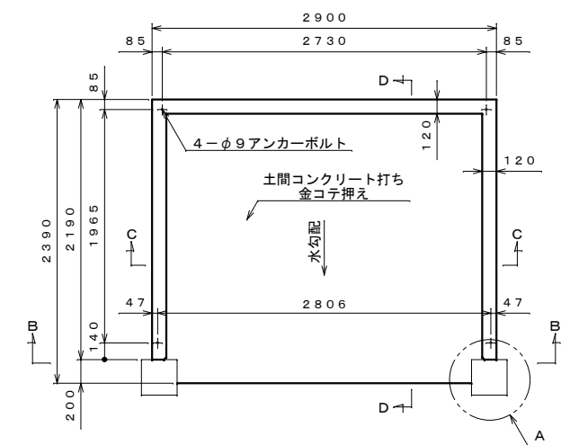
基礎伏せ図 S=1:40
