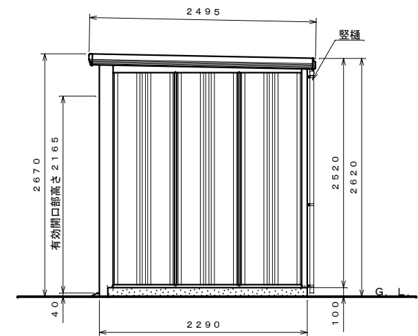
側面図 S=1:40
