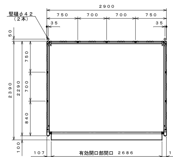
平面図 S=1:40
