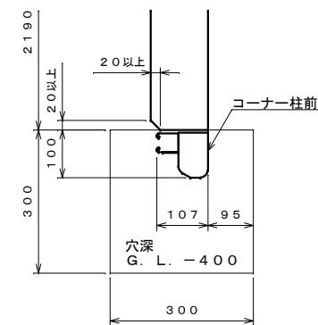
A部詳細図 S=1:10
