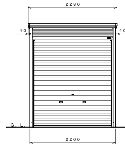
正面図 S=1:40
