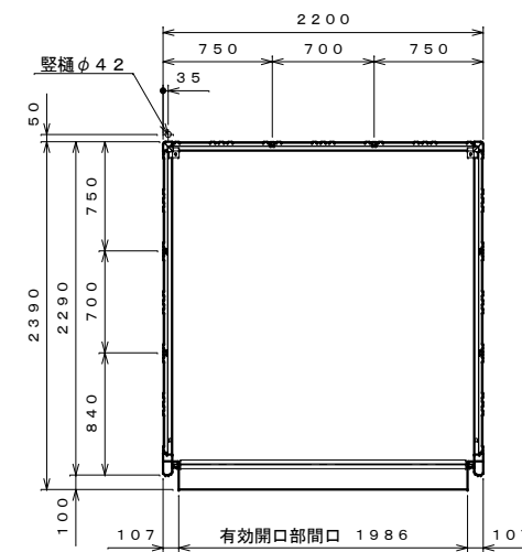
平面図 S=1:40
