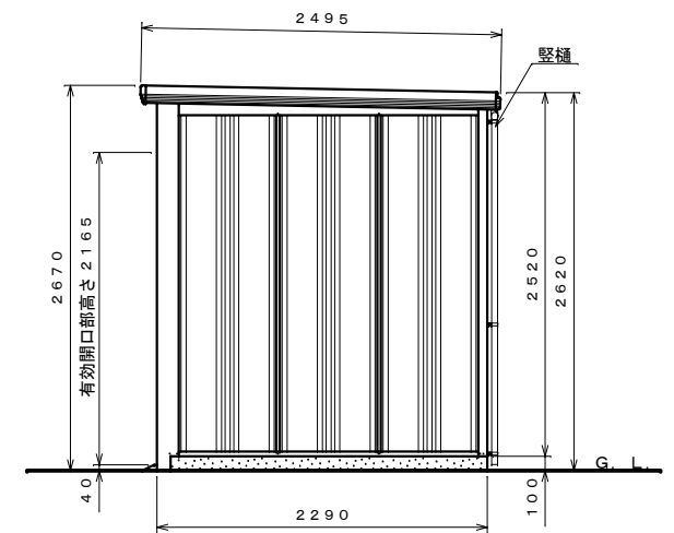
側面図 S=1:40
