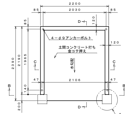
基礎伏せ図 S=1:40
