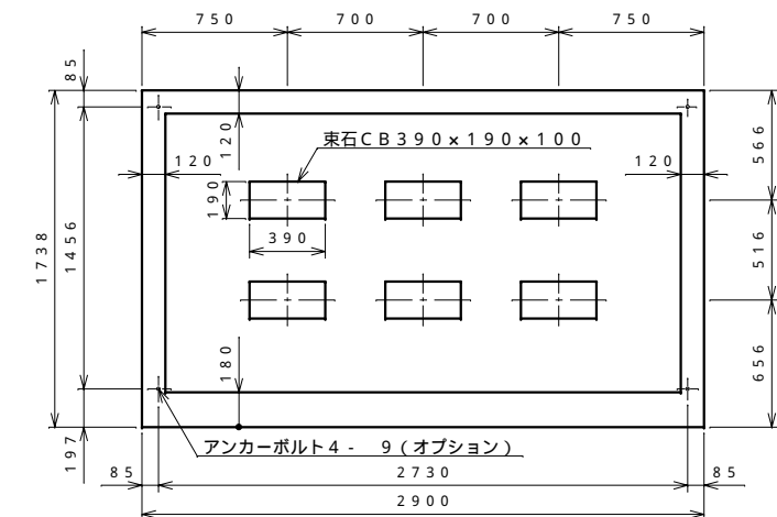
基礎伏図 S = 1 : 30
