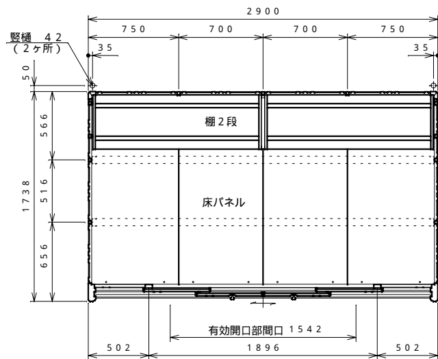
平面図 S = 1 : 30
