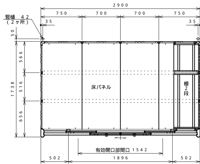
平面図 S = 1 : 30
