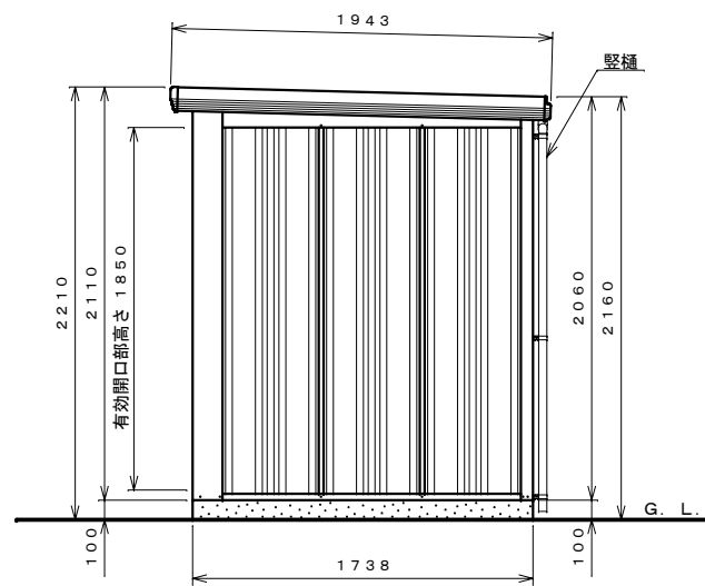
側面図 S=1:30
