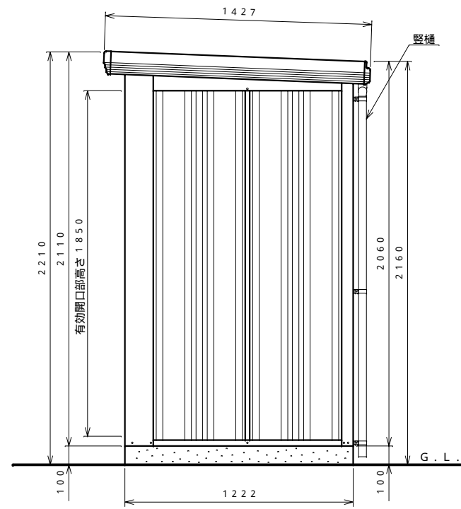
側面図 S = 1 : 20
