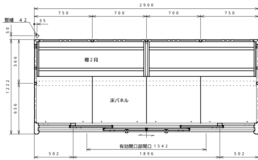
平面図 S = 1 : 20
