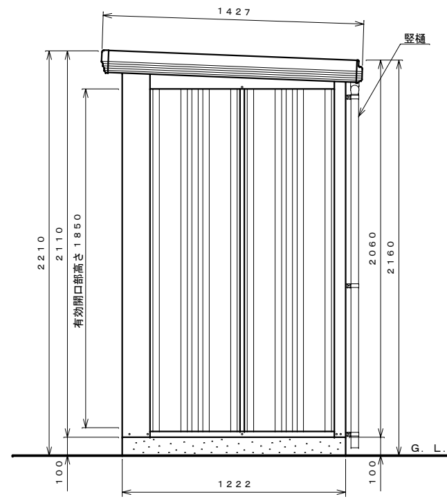
側面図 S=1:20
