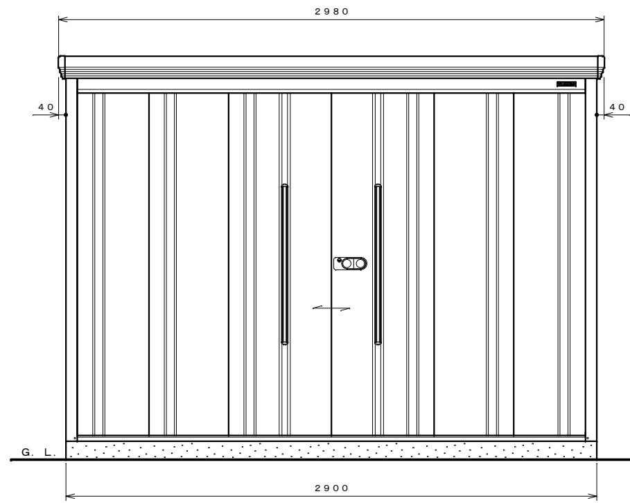
正面図 S=1:20
