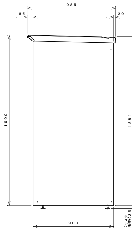
右側面図
