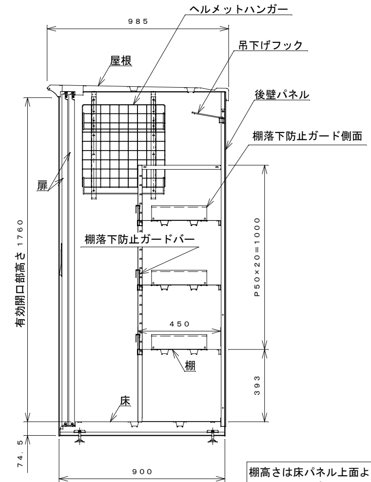
側面断面図
