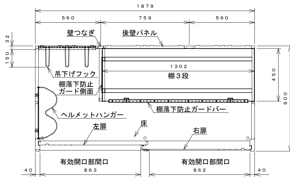
平面断面図
