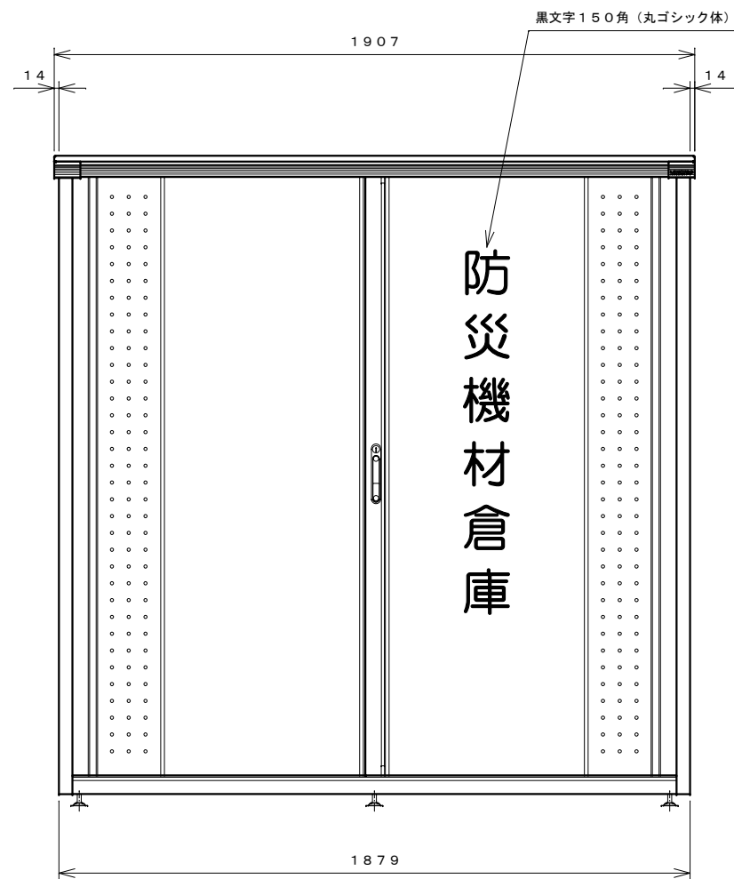
正面図
