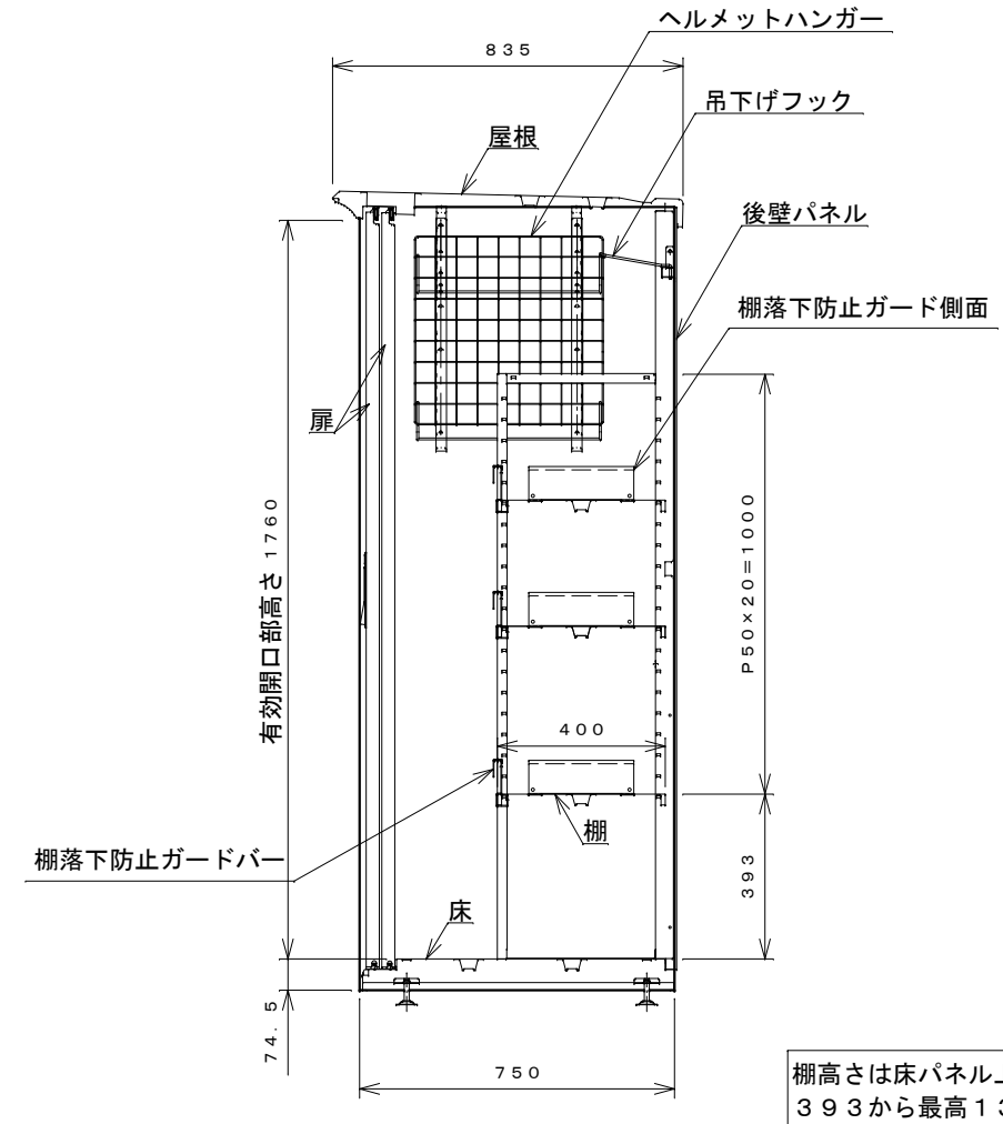
側面断面図
