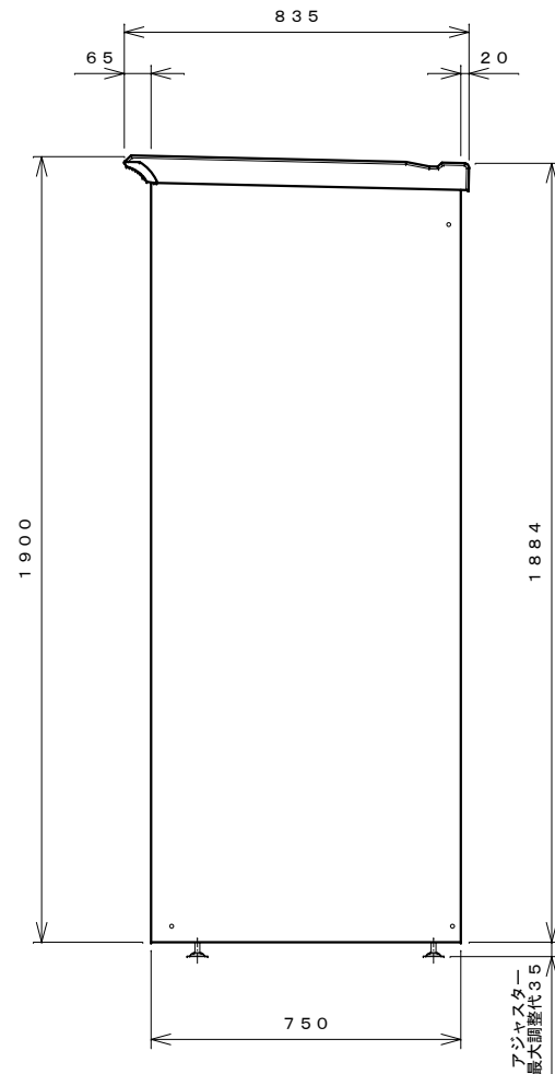
右側面図
