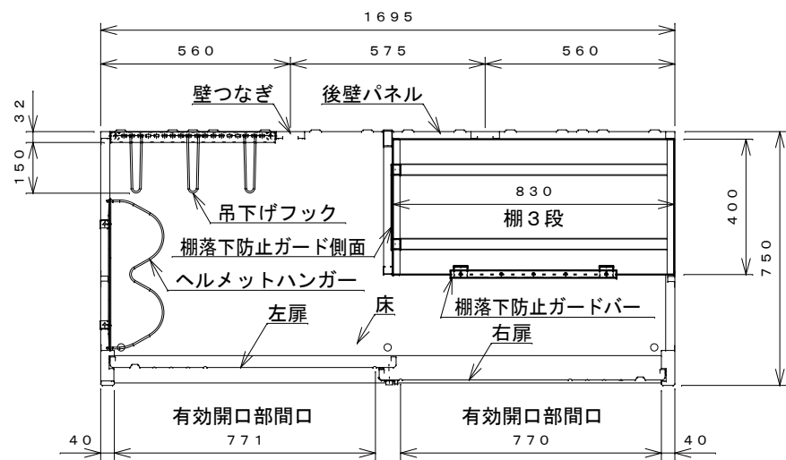
平面断面図
